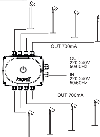
Bloom Mini Bollard HUB.700.001.ND MAX 8 pz. 700mA Not Dimmable
