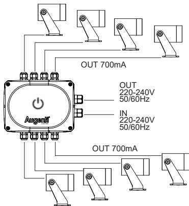
Bloom Mini HUB.700.001.ND MAX 8 pz. 700mA Not Dimmable
